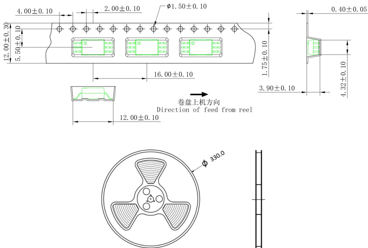
图 24 编带包装示意图 Figure 24- Taping Packing Schematic
