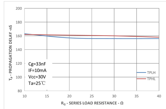
图 16 T_P - R_g 特性曲线
