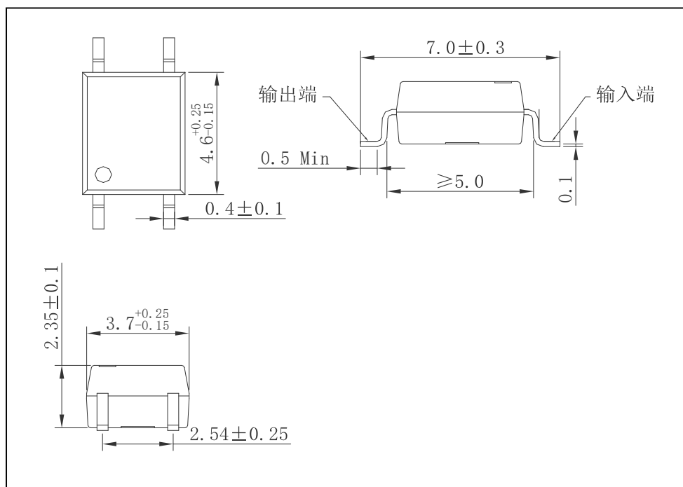
图 4 HSSR-S1A08-2 外形尺寸
