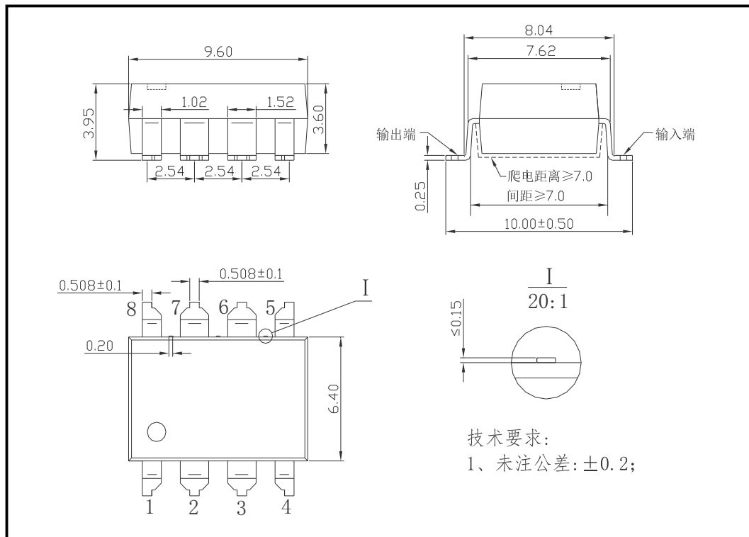
图 4 HSSR-DA05-2 外形尺寸 Figure 4- The dimensions of HSSR-DA05-2
