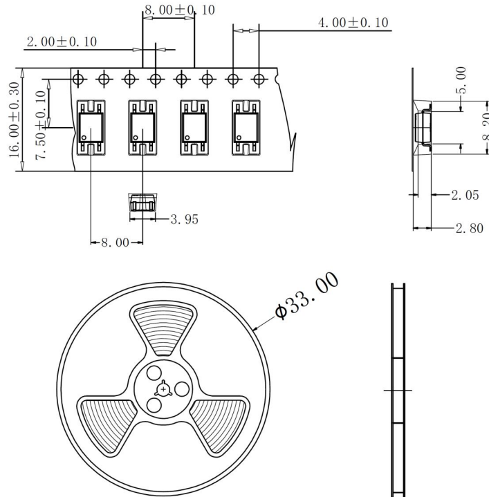
图 5 编带包装示意图 Figure 5- Taping Packing Schematic
