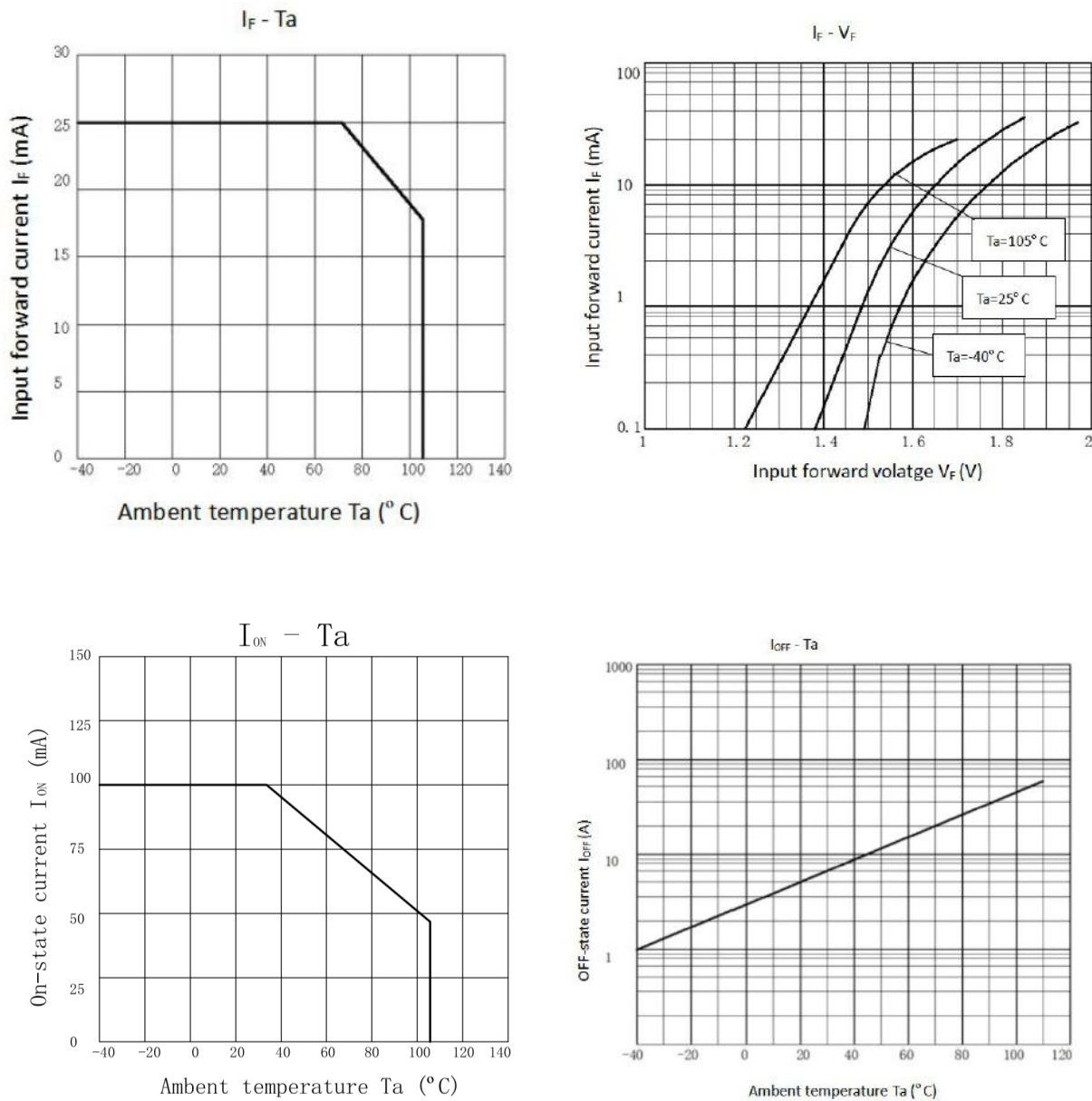
图3 特性曲线
