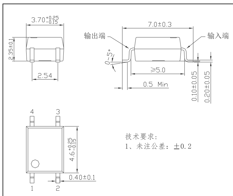
图 4 HSSR-S1A04-2 外形尺寸
