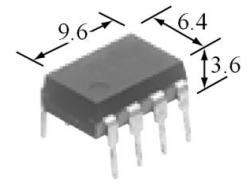
图 1 产品 Figure 1-Product
