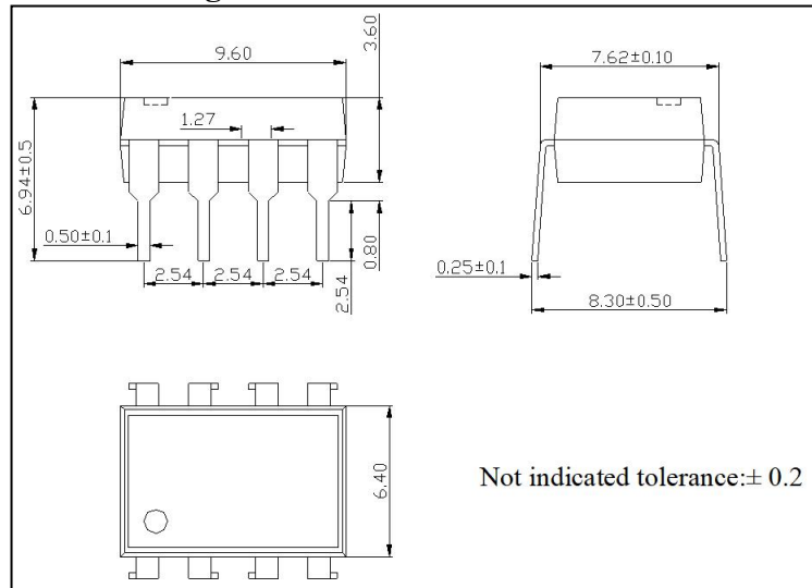
图 3 HPC300 外形尺寸
