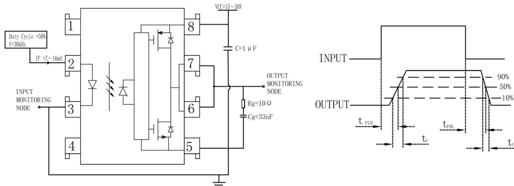
图 3 t_{PHL}, t_{PLH} 测试方法 Figure 3- The test method of t_{PHL}, t_{PLH}
