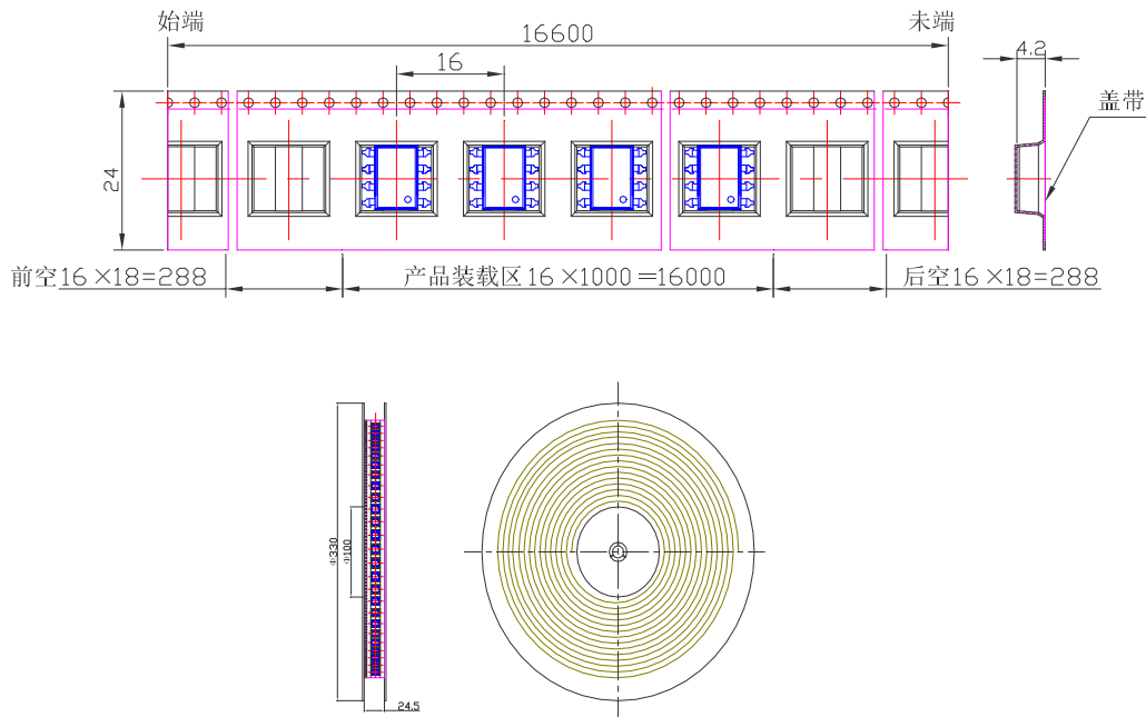
图 8 编带包装示意图
