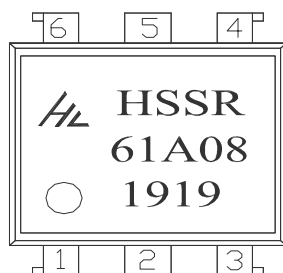
图 6 产品印章 Figure 6- Marking
