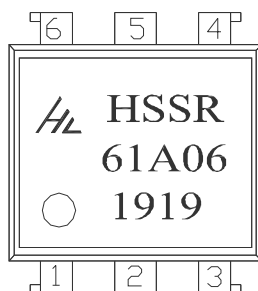
图 6 产品印章 Figure 6- Marking
