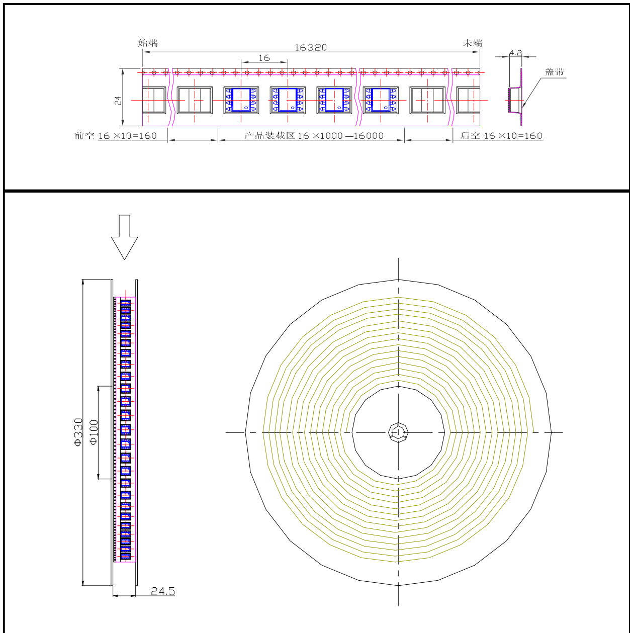
图 7 编带包装示意图 Figure 7- Taping Packing Schematic
