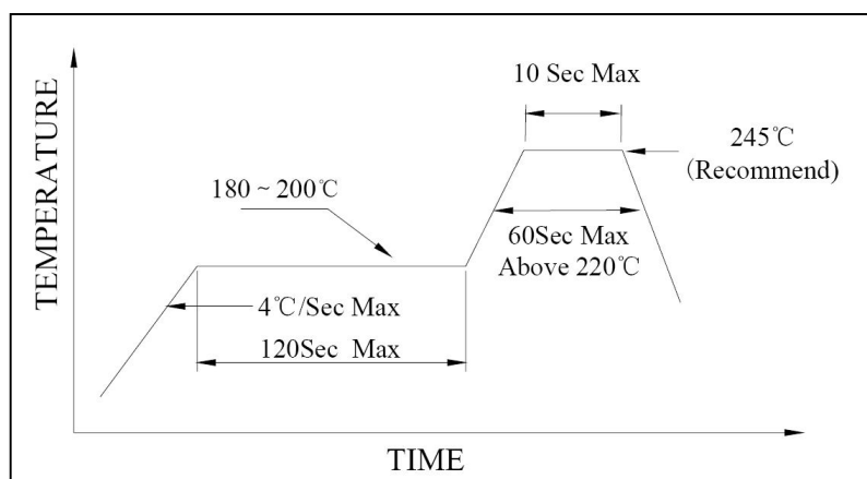
图9 回流焊参数
