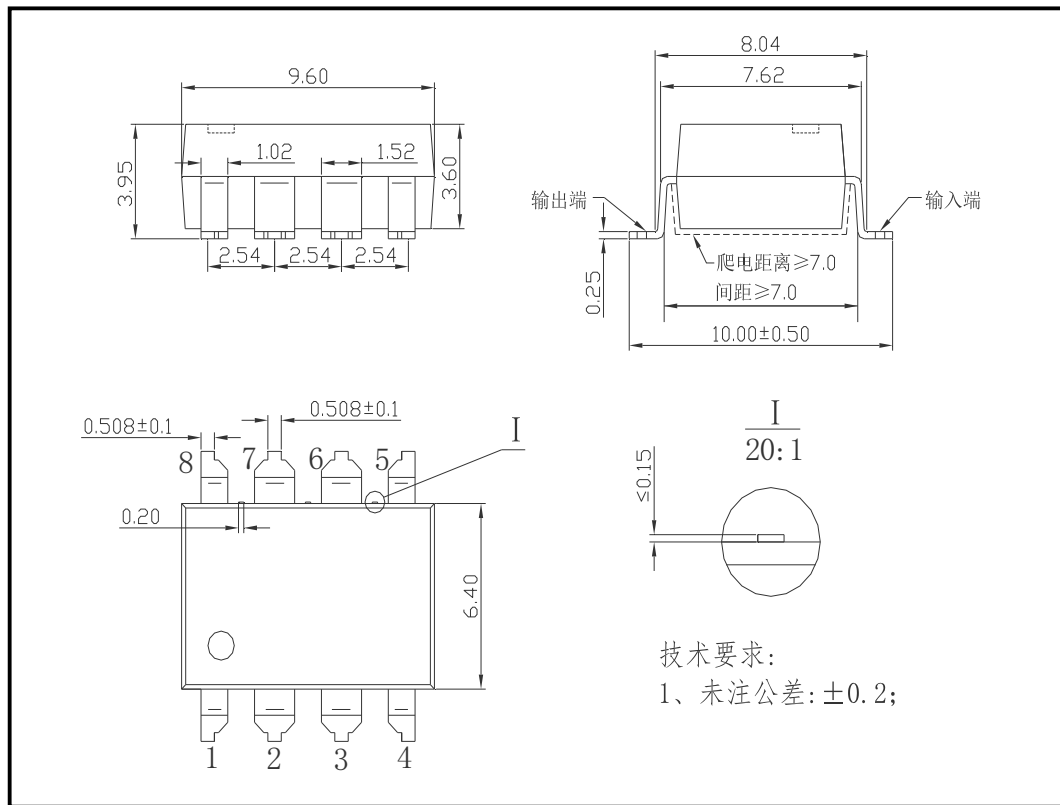
图 4 HSSR-DA01-2 外形尺寸
