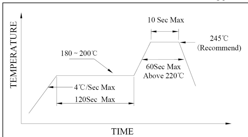
图 10 回流焊参数
