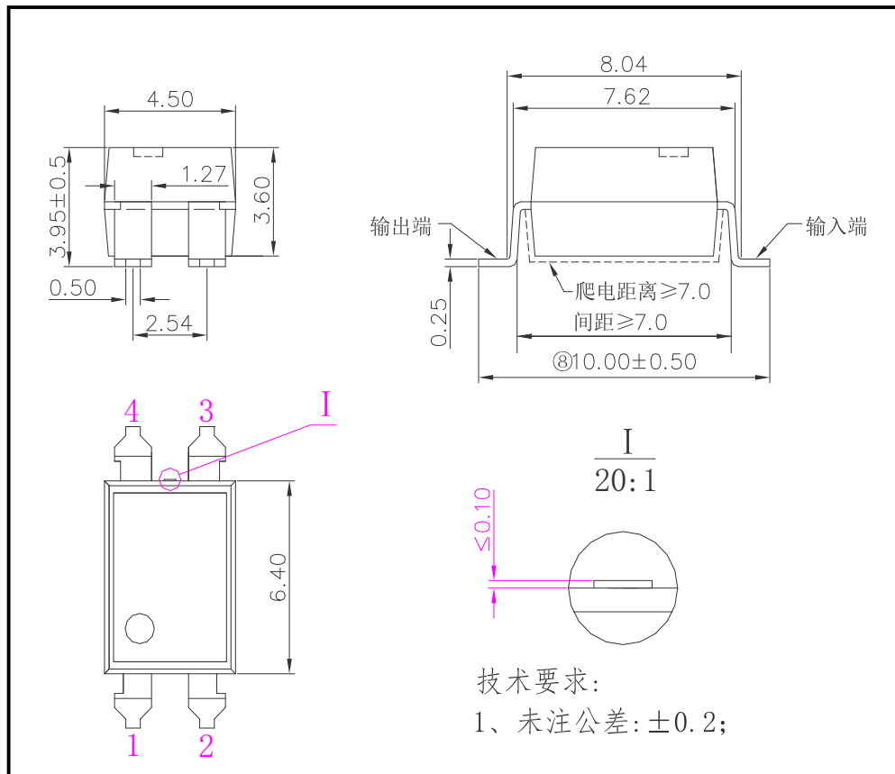
图 4 HSSR-41A06-2 外形尺寸
