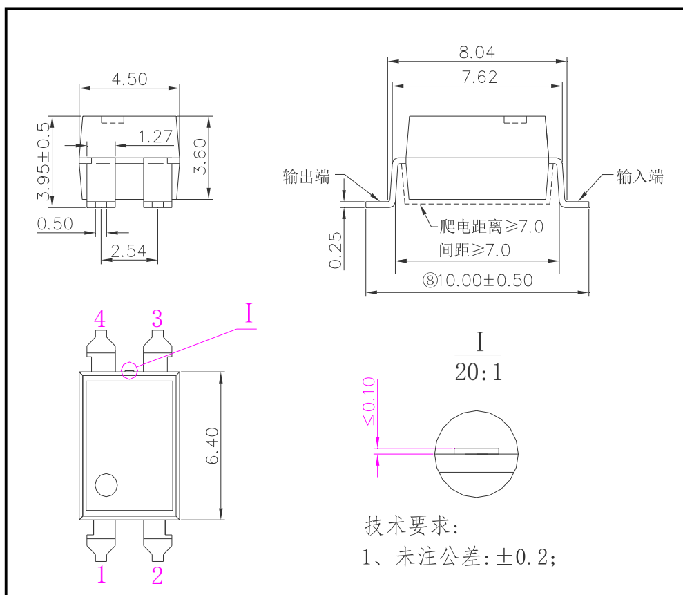
图 4 HSSR-41A04-2 外形尺寸
