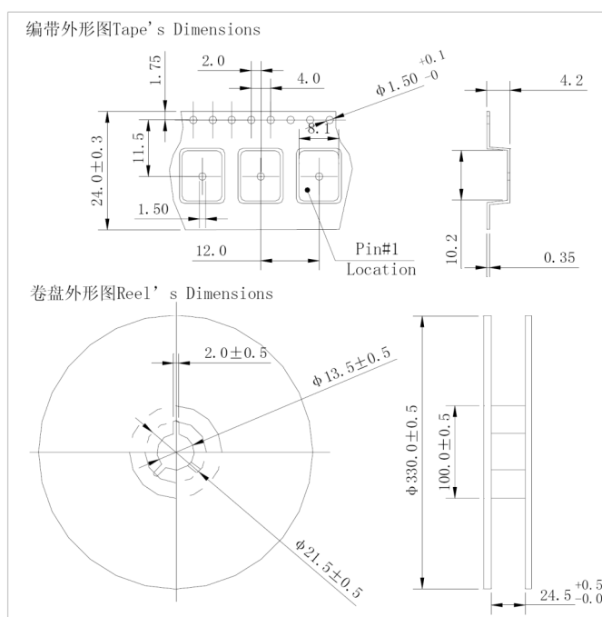
图 5 编带包装示意图
