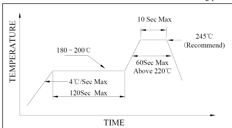
图 7 回流焊参数
