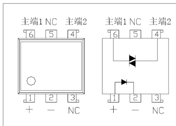
图 3 电原理图
