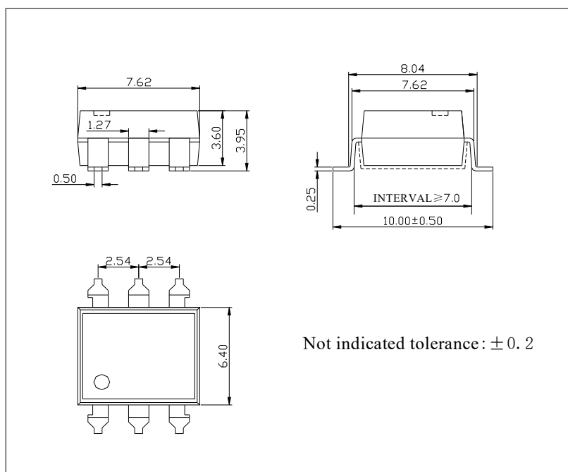
图 2 外形尺寸
