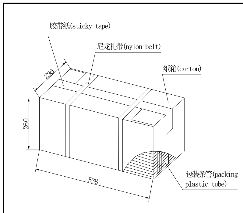
图 5 条管外包装
