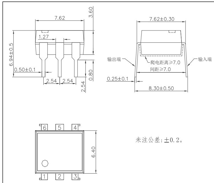
图 2 外形尺寸
