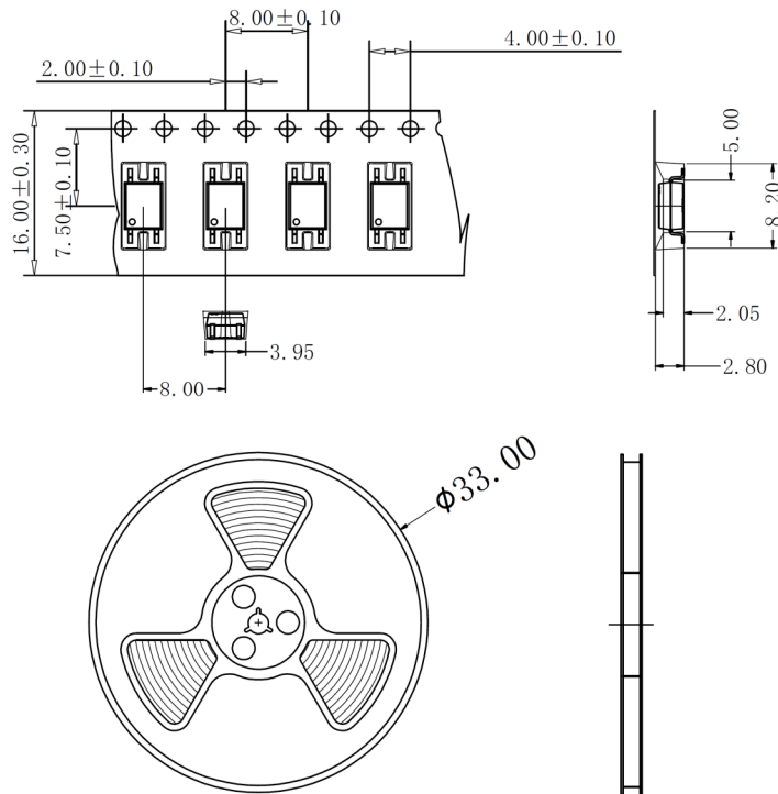
图 6 编带包装示意图
