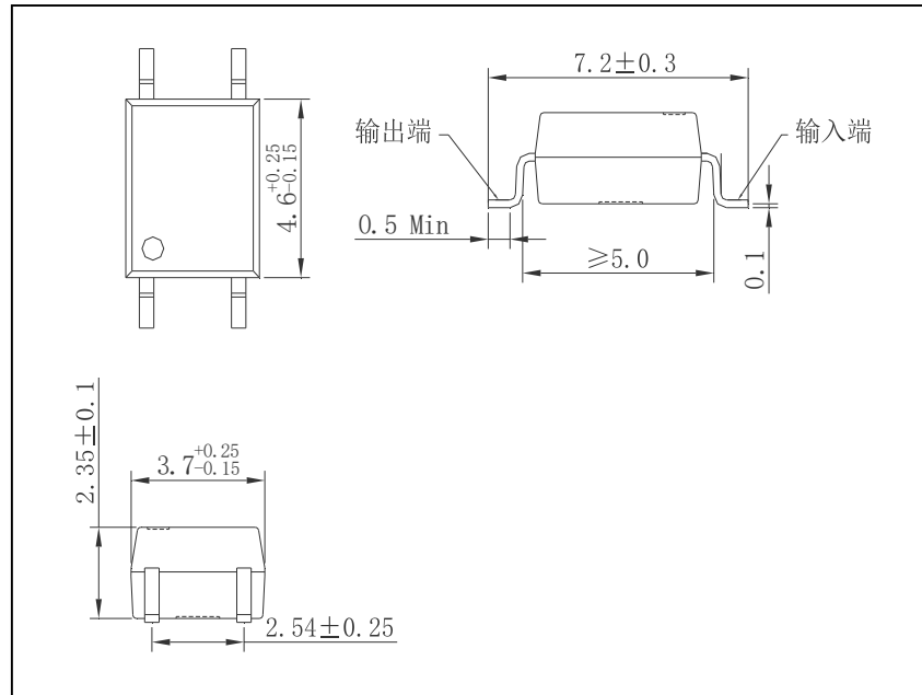
图 4 HSSR-S1A01-2 外形尺寸
