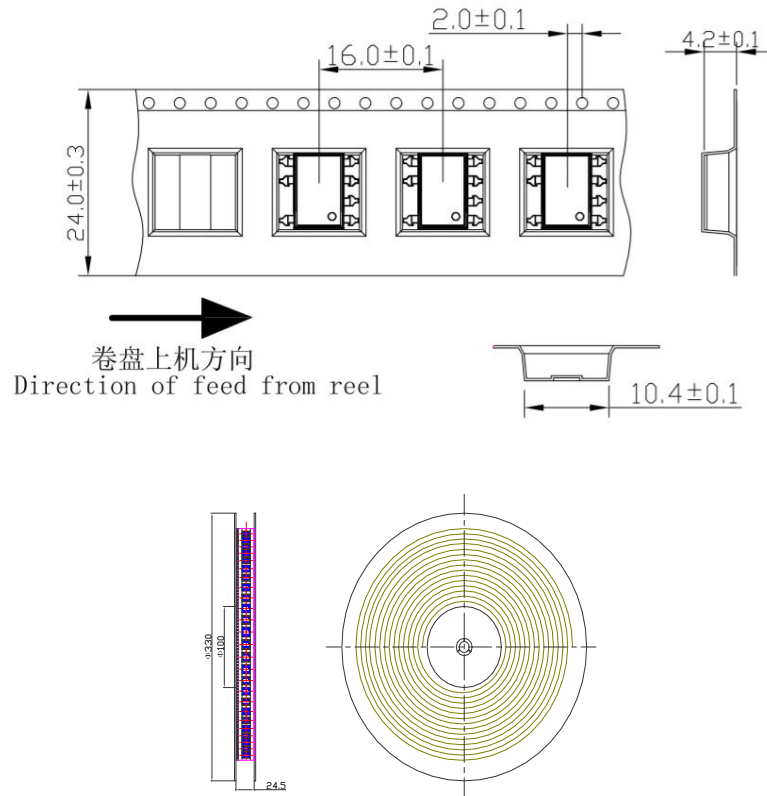
图 7 编带包装示意图
