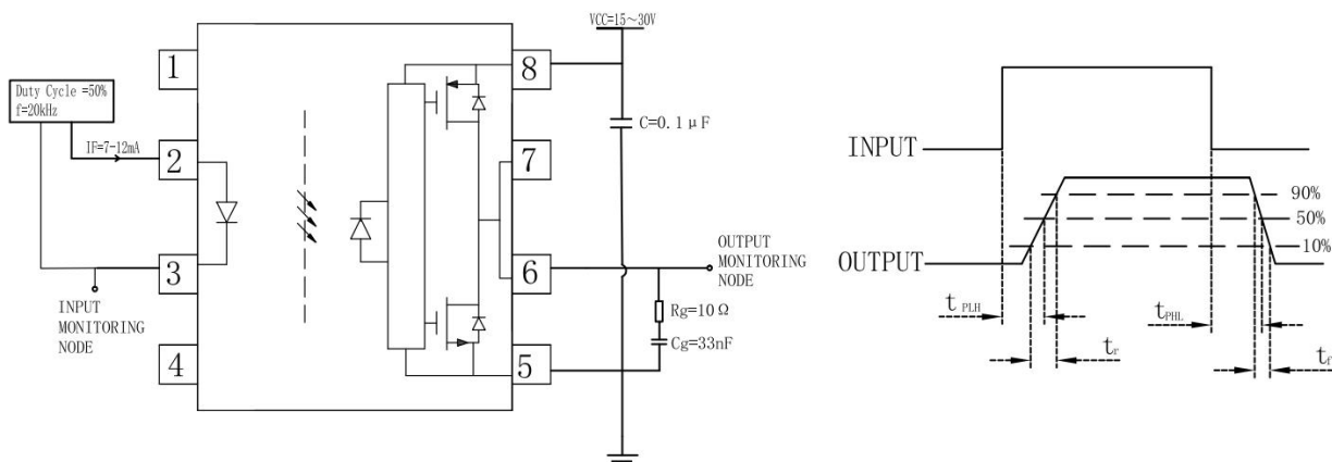
图 11 t_{PHL} , t_{PLH} 测试方法 Figure 11- The test method of t_{PHL} , t_{PLH}
