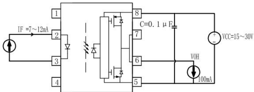
图 9 VOH 测试电路
