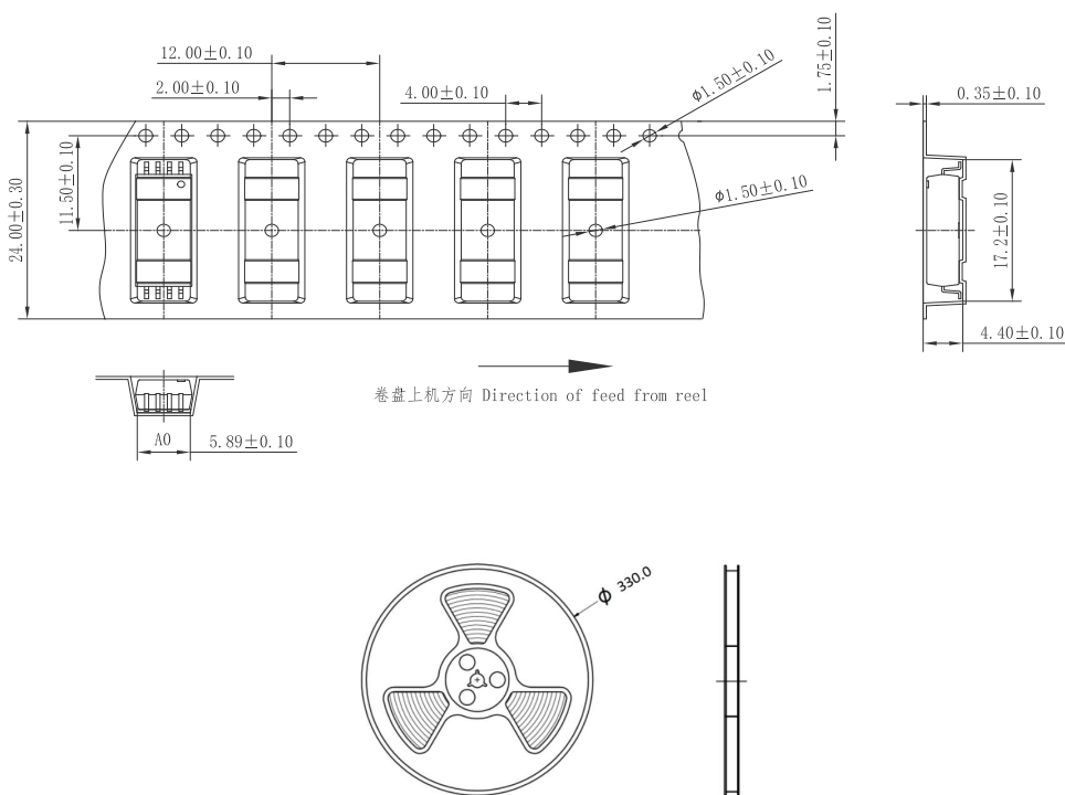
图 14 编带包装示意图
