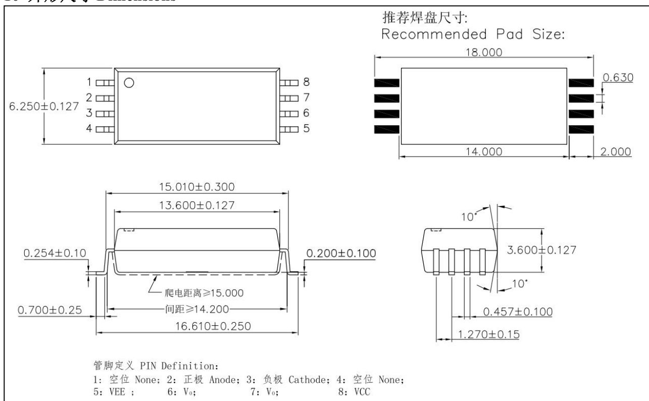
图 12 HGD313H 外形尺寸 Figure 12- The dimensions of HGD313H
