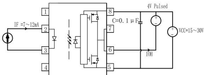
图 7 I_{OH} 测试电路
