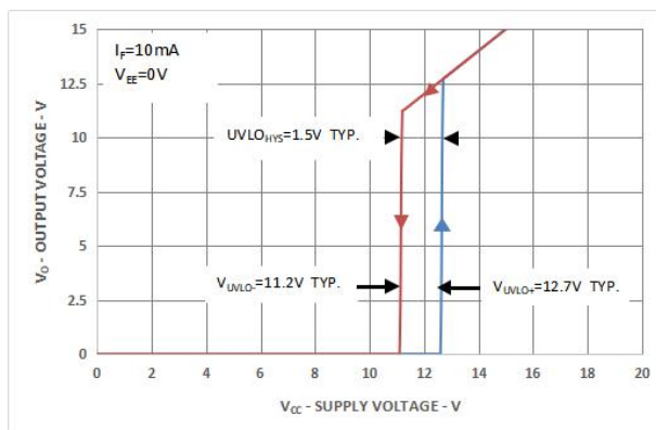
图 5 低压双锁特性曲线
