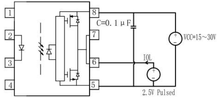
图 8 IOL 测试电路
