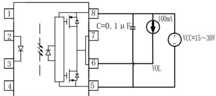
图 10 VOL 测试电路
