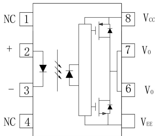
图 2 电原理图
