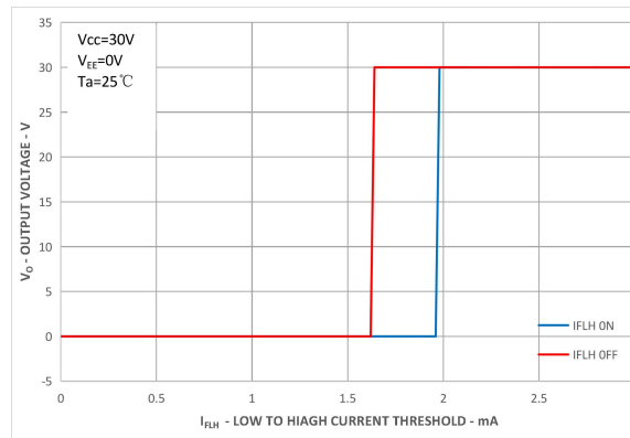
图 6 I_{FLH} 滞后特性曲线
