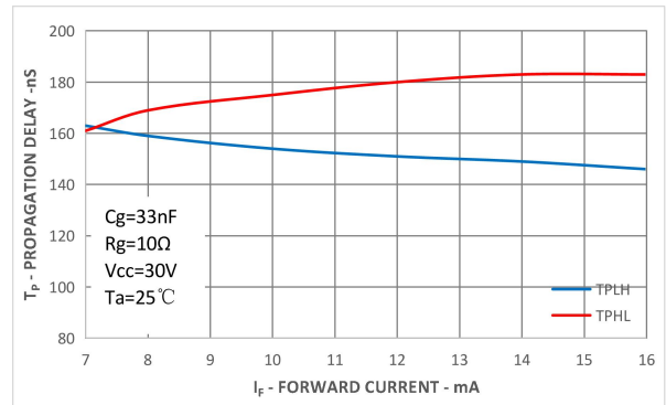
图 14 T_P - I_F 特性曲线
