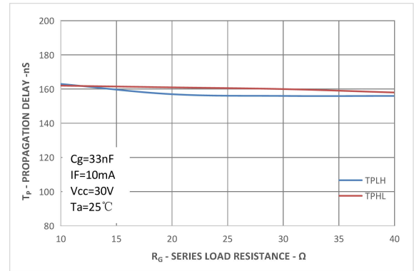
图 16 T_P - R_g 特性曲线
