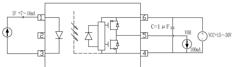
图 19 V OH 测试电路
