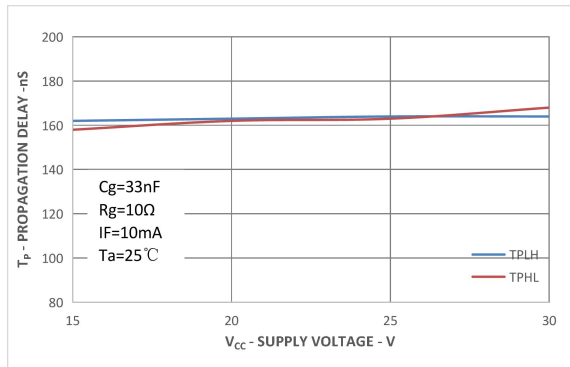
图 13 T_P - V_{CC} 特性曲线
