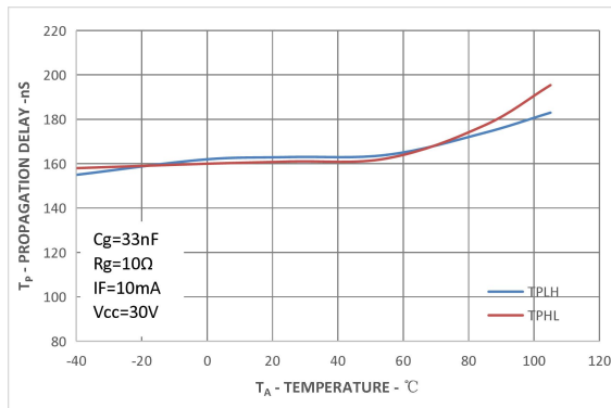
图 15 T_P - T_A 特性曲线
