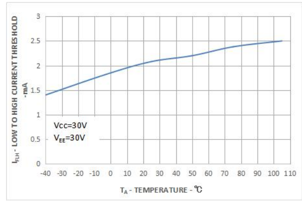
图 12 I_{FLH} - T_A 特性曲线
