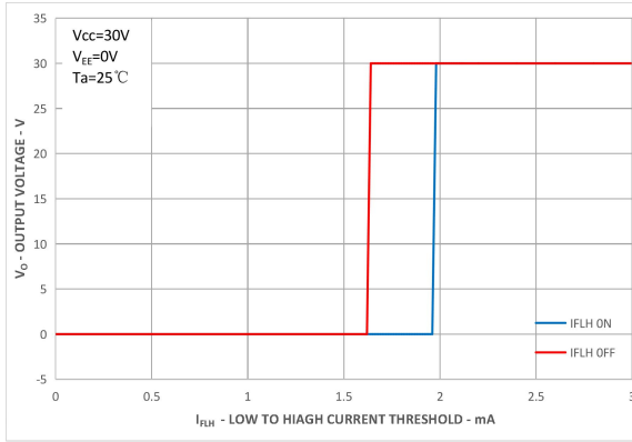
图 11 I_{FLH} 滞后特性曲线
