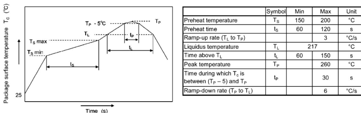
图 7 回流焊参数
