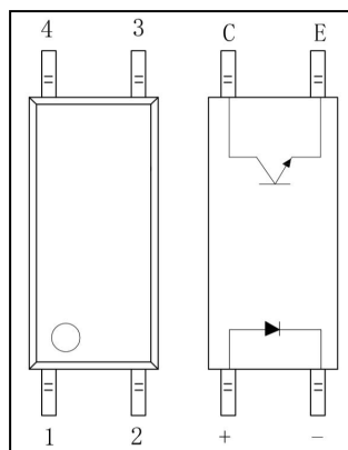
图 3 电原理图 Figure 3-Schematic
