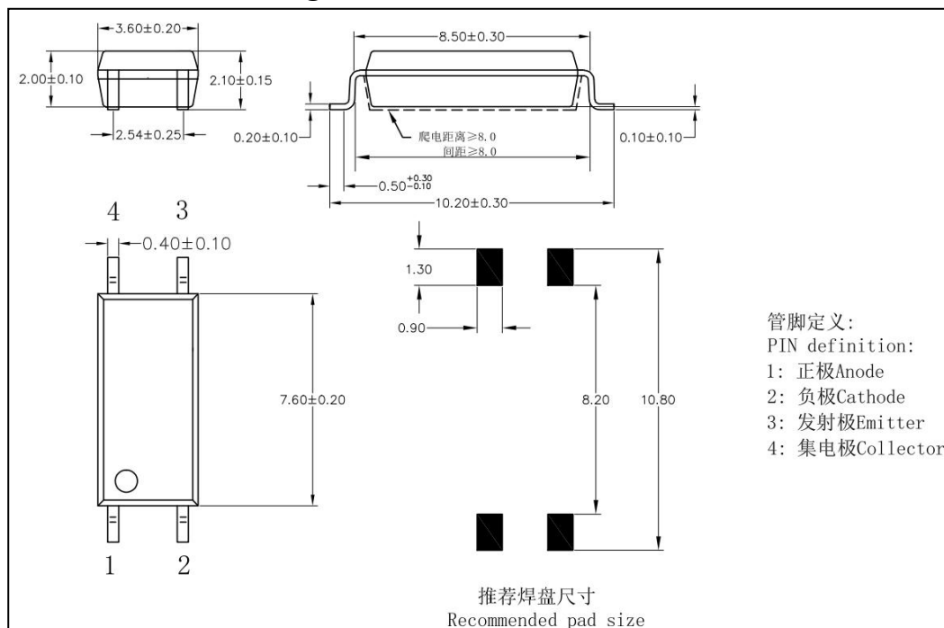
图 4 HPC101× 外形尺寸
