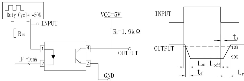
图 2 t_{on} , t_s , t_{off} 测试方法
