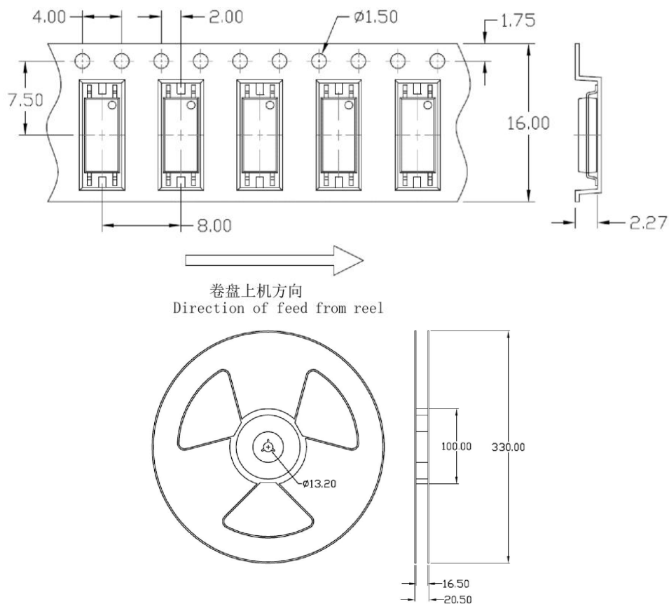
图 6 编带包装示意图
