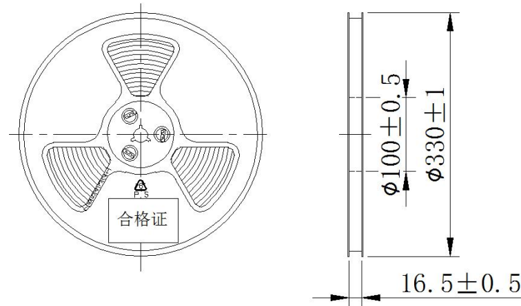
图 7 编带包装示意图 Figure 7- Taping Packing Schematic
