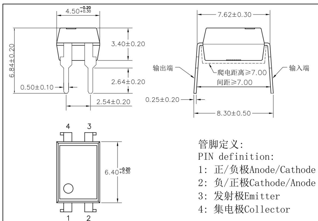
图 3 HPC814× 外形尺寸
