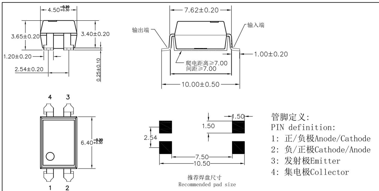
图 4 HPC814×-2 外形尺寸 Figure 4- The dimensions of HPC814×-2
